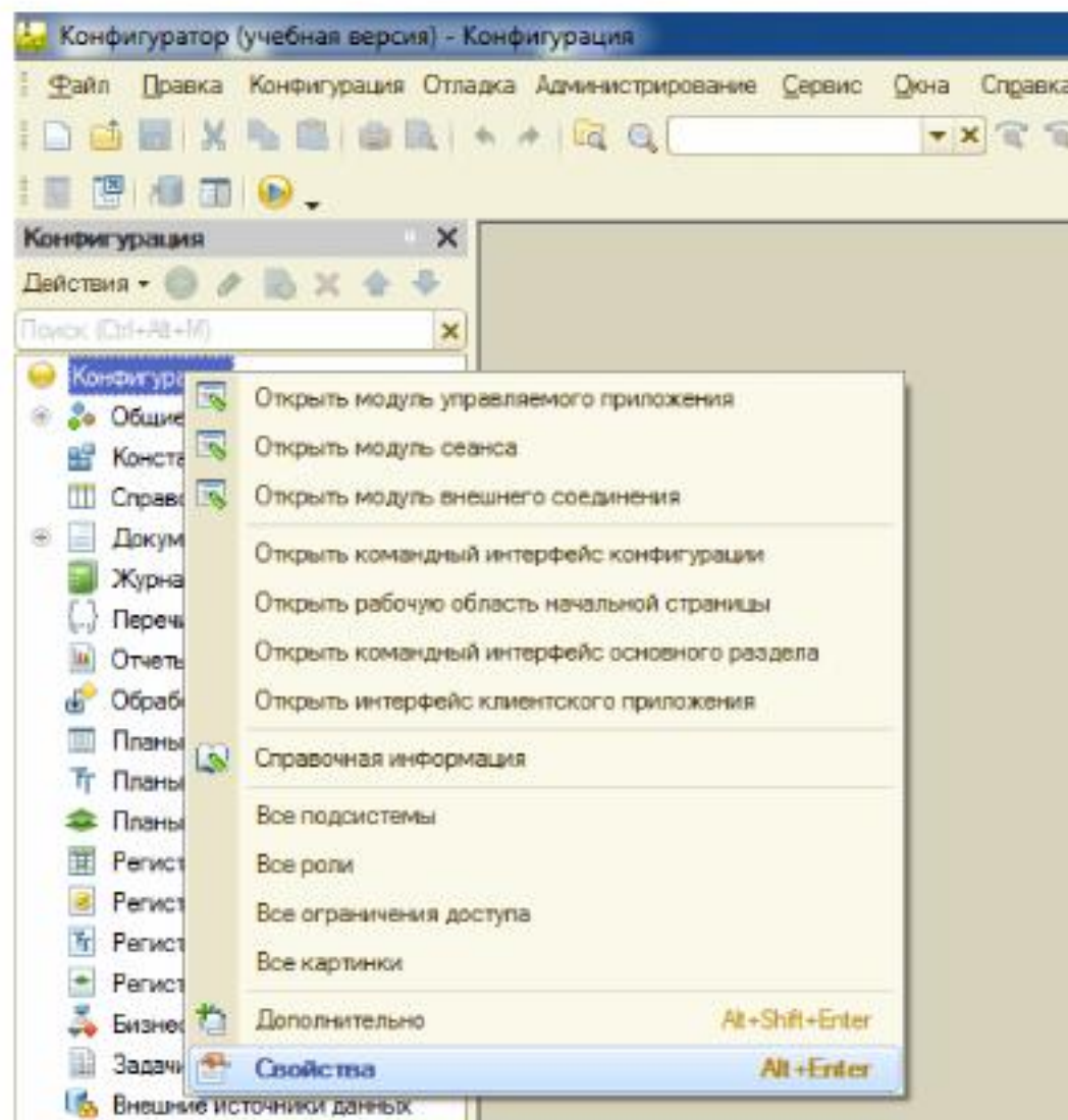
Рис. 6. Свойства конфигурации
