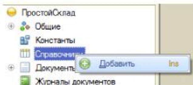
Рис. 8. Добавление справочника
