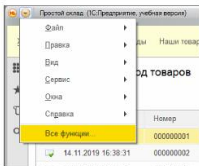
Рис. 46. Все функции
