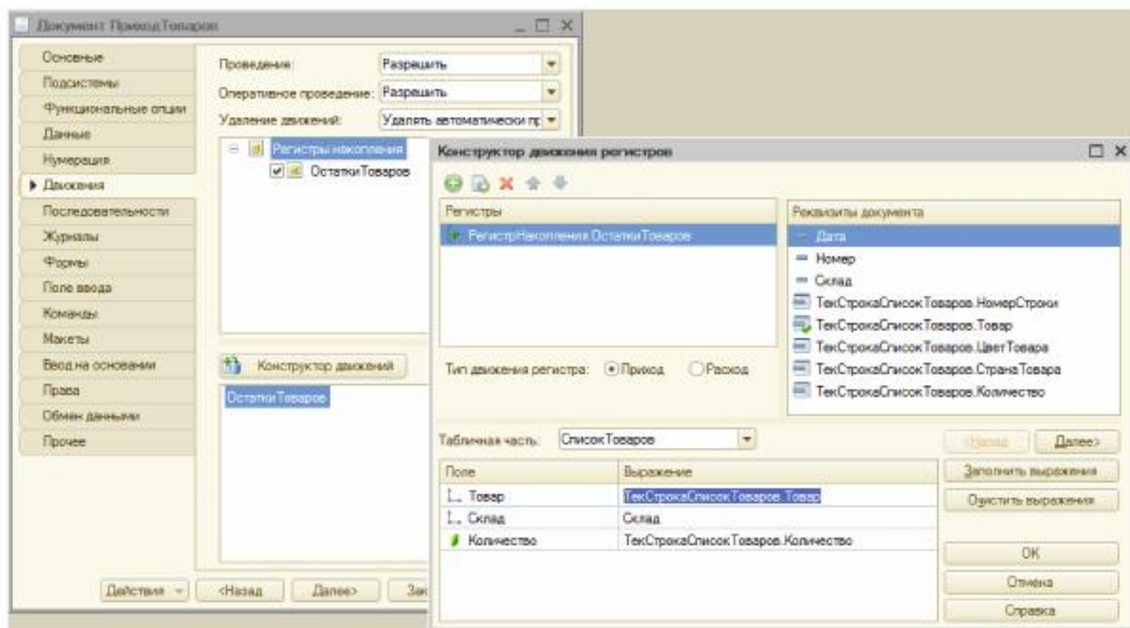
Рис. 39. Конструктор движений
